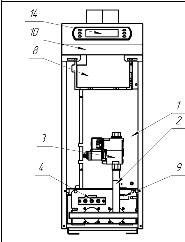
Рисунок 1 – конструкция котла КОВ-СК(В)Се
