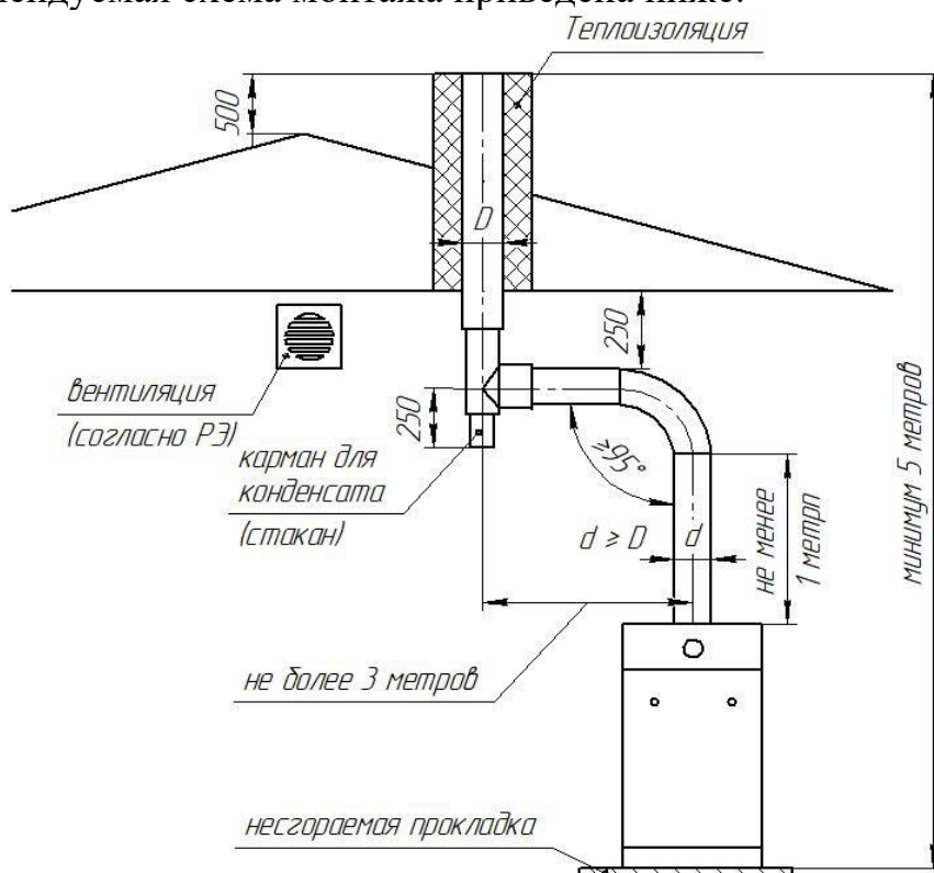
Рисунок 8 – Схема монтажа дымохода
